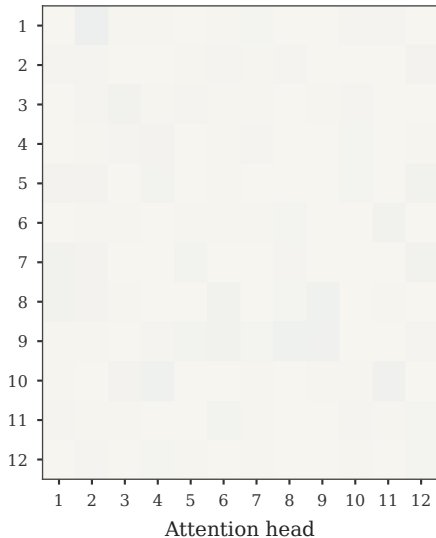
Base GPT-2
